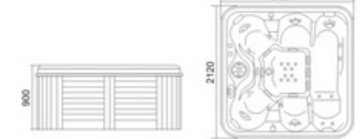
KB-209 2120x2120x900mm
