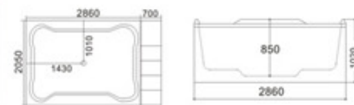
KB-206 3560x2050x1020mm
